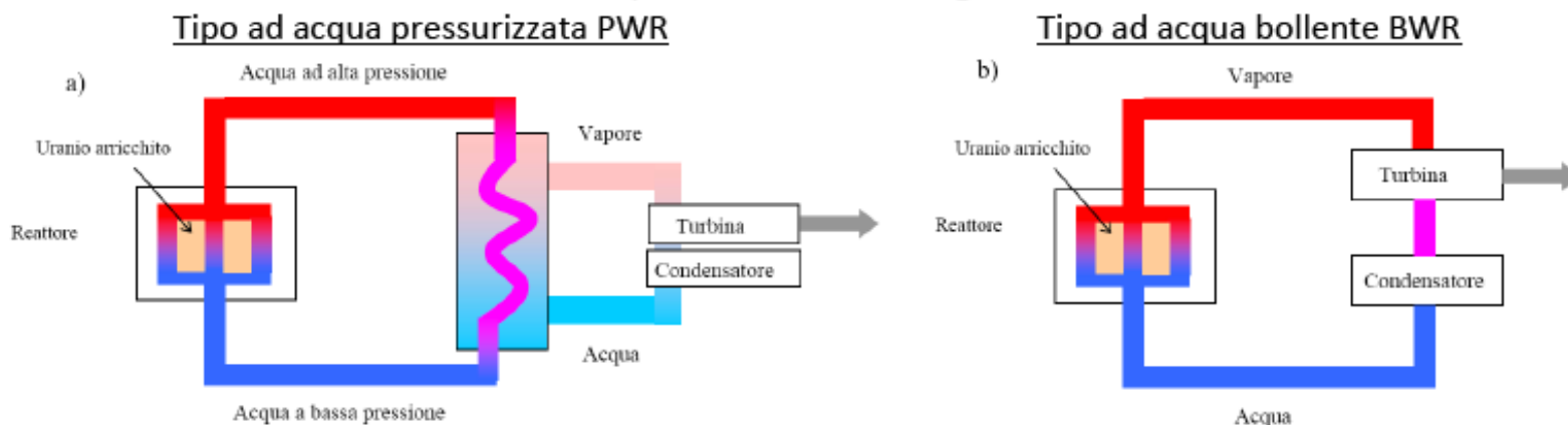
Schema di impianto nucleare di II a generazione
